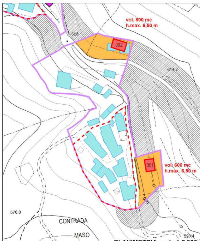
PLANIMETRIA scala 1:2.000
